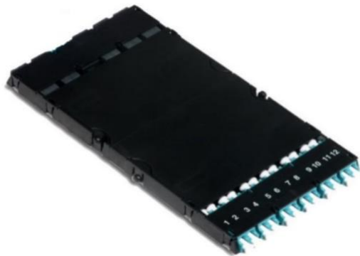
Fig. 2: HX Base-12 MPO Breakout
